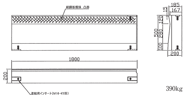
零段差 斜 300用(右・左)
