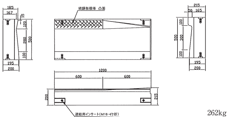
零段差 斜 300用(右・左)
