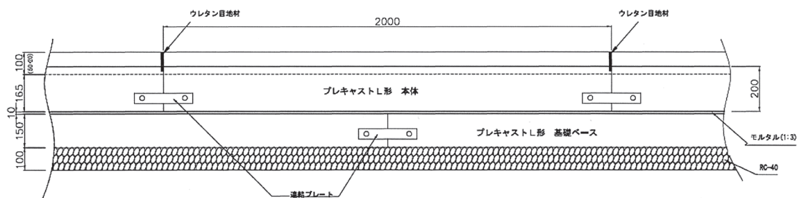
敷設図構造図 (正面)
