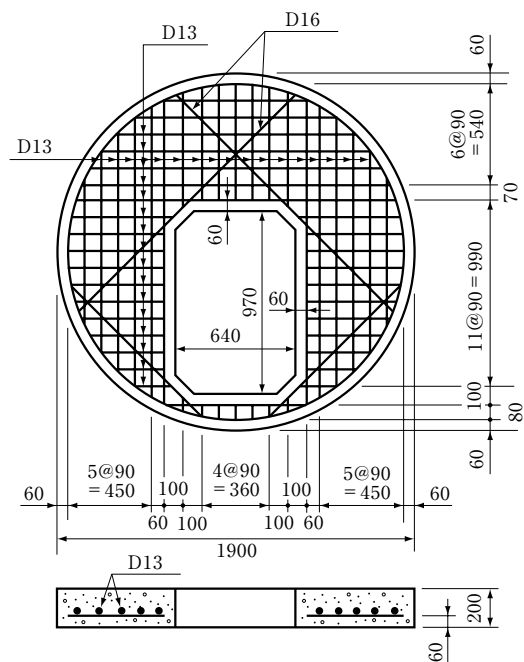
頂版 (100～200mm)
