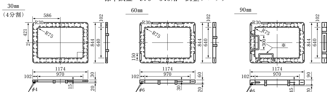
標準鉄蓋 970×640用 調整ブロック
