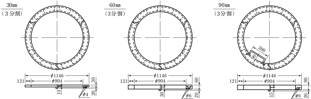
人孔室鉄蓋 \phi 900 用 調整ブロック 空気弁室用
