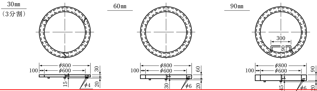
人孔室鉄蓋 \phi 900 用 調整ブロック 空気弁室用
