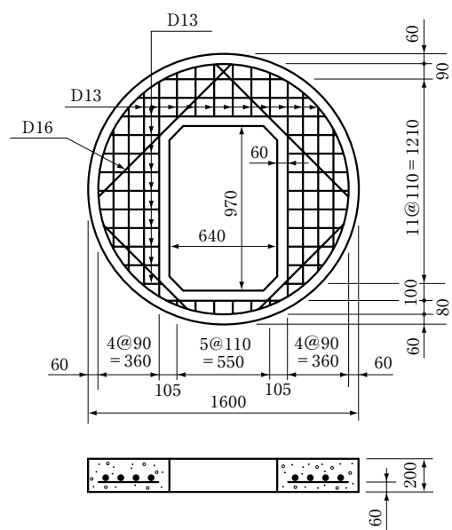
頂版 (75mm)
