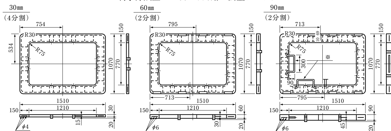
制水弁鉄蓋 1200×770用 調整ブロック
