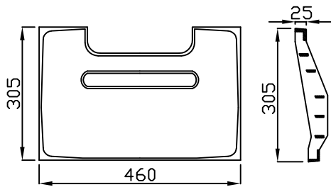
雨水桧 250用マーク無
