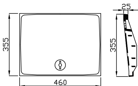
汚水桧 300用マーク無
