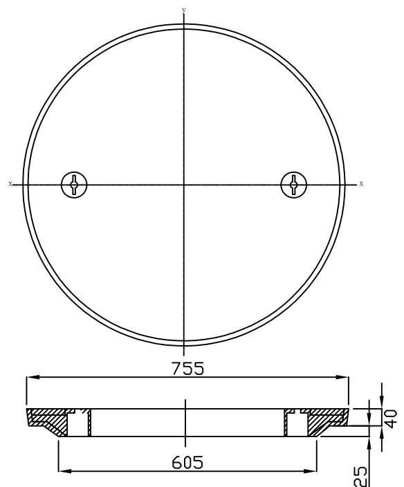
汚水柵 700用 マーク無
