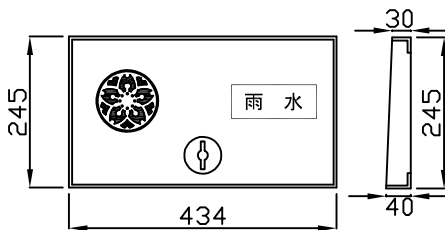
LU縁塊 300用
