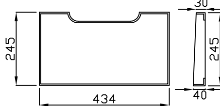
LU縁塊 300用
