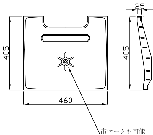
雨水枡 350用都マーク
