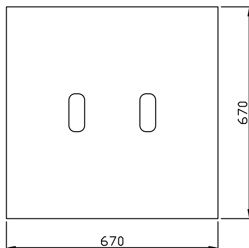
D型 600用
