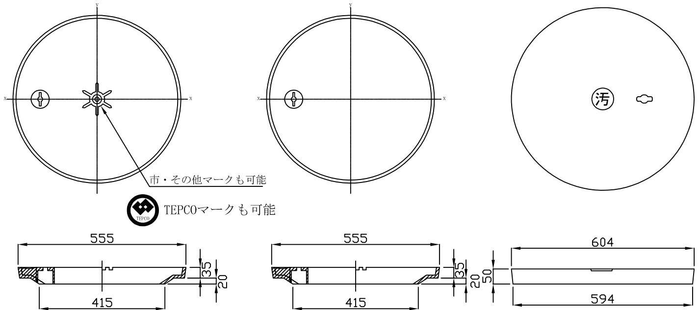
汚水枡 500用都マーク
