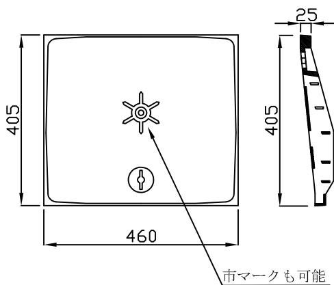
汚水枡 350用都マーク
