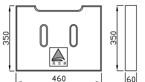
L形集水枡 300用足立区型
