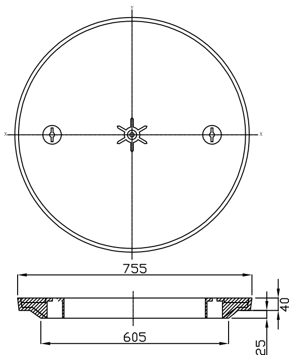
汚水柵 700用 都マーク
