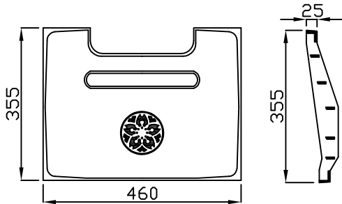
雨水桧 300用都桜マーク
