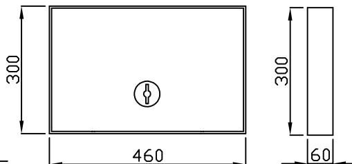
L形集水閉塞蓋 250用
