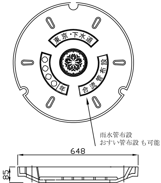
歩道用人孔ふた桜マーク
