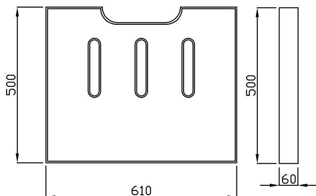
街きょ枡 206型
