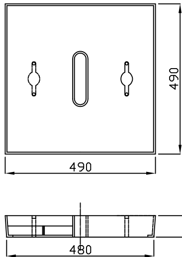
U形用集水桝(装鉄製) (取手金具付)
