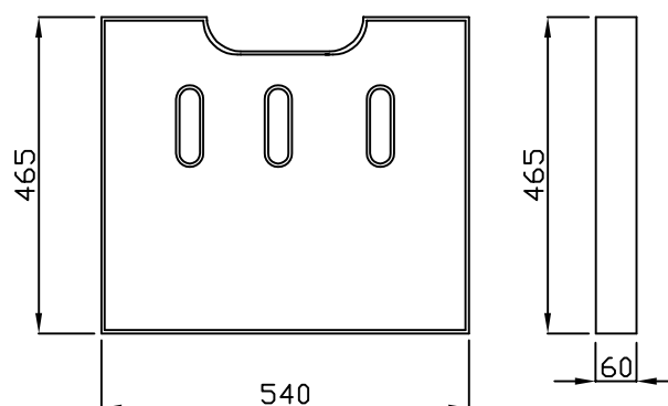
街きょ枡 1種
