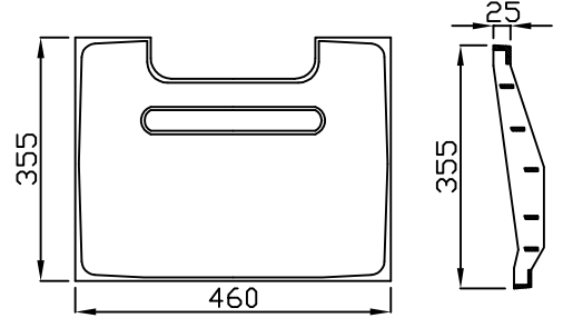
雨水桧 300用マーク無
